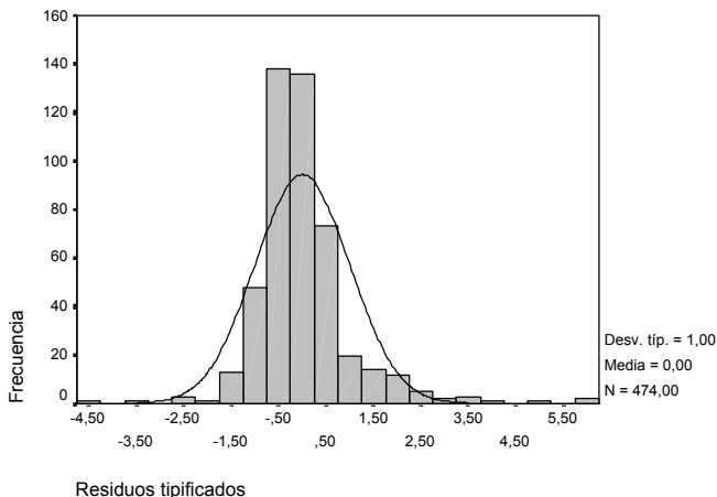
Figura 18.9. Histograma de los residuos tipificados.
