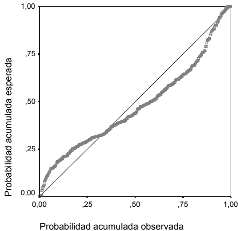
Figura 18.10. Gráfico de probabilidad normal de los residuos.
