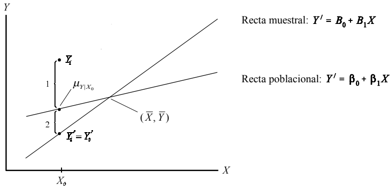
Figura 18.14. Tipos de error en los pronósticos de la regresión.
